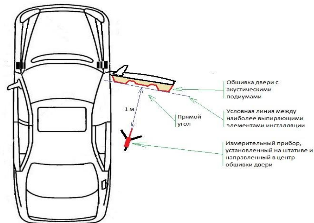
Рисунок 3. Расположение измерительного оборудования во время финального замера.
