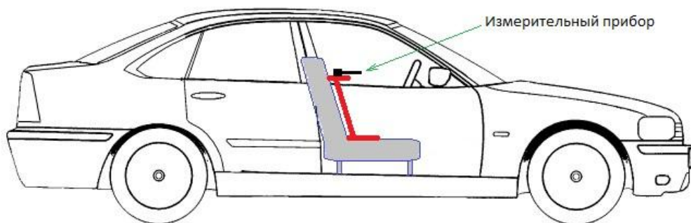
Рисунок 1. Расположение измерительного оборудования во время квалификационного замера классов Фронт 1, 2 и 3.
