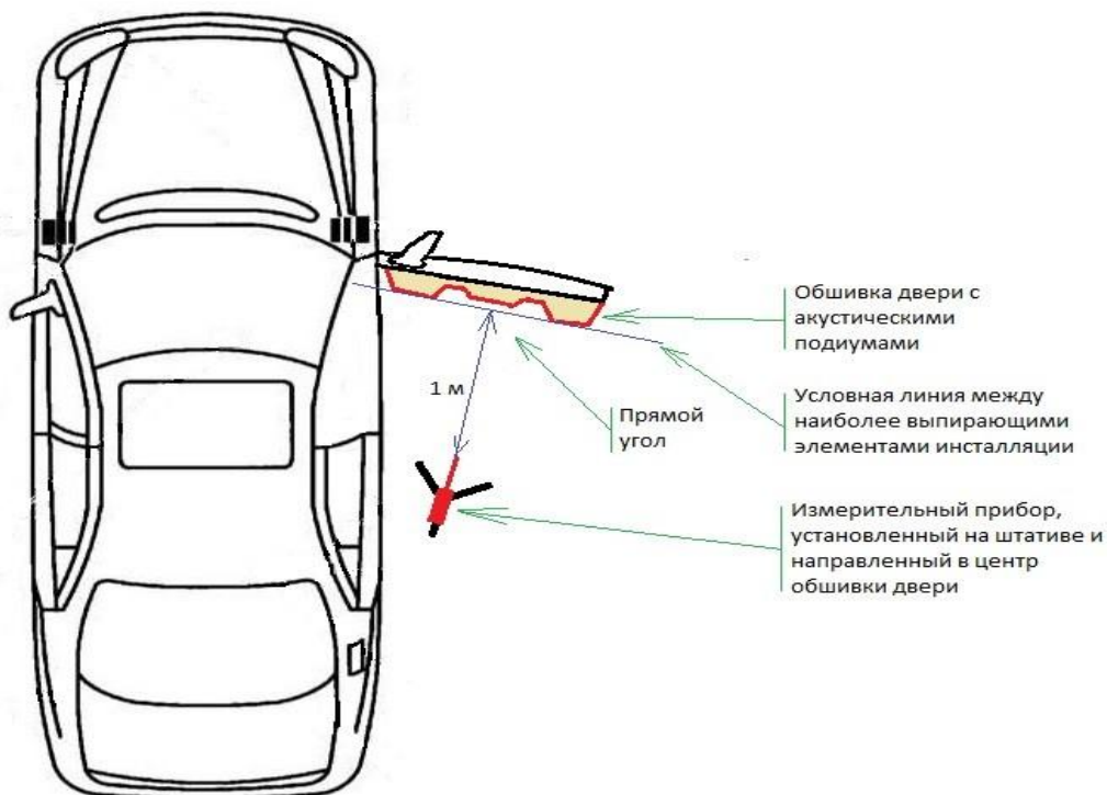
Рисунок 3. Расположение измерительного оборудования во время финального замера.
